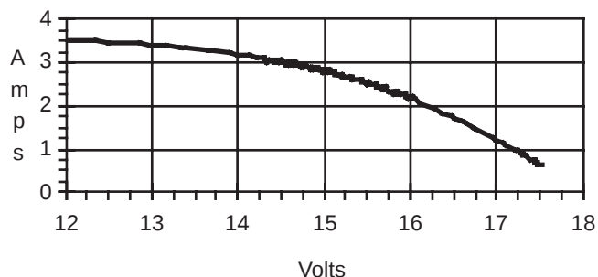
Solarex MSX60
