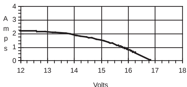
ARCO 16-2000
