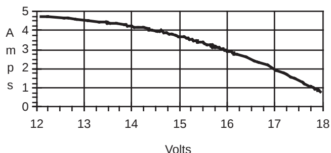
Siemens PC4JF
